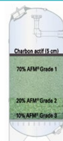
Stratification du filtre avec AFM®
